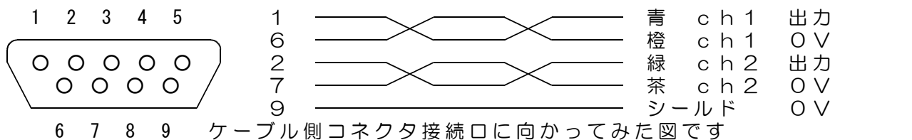
9DS-500 標準ケーブル長 50cm
