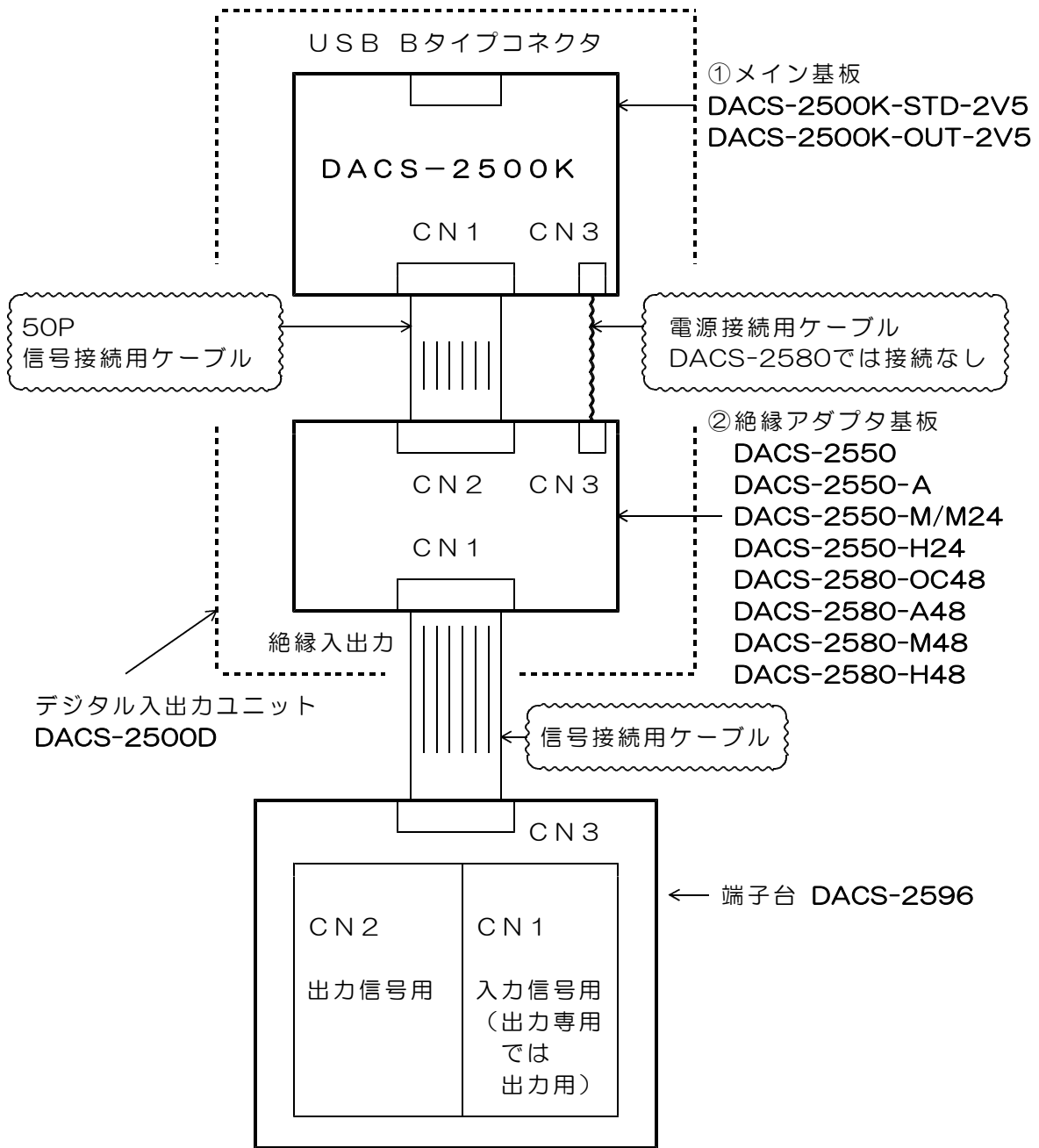
図1 DACS-2500ESシリーズ 内部接続図
