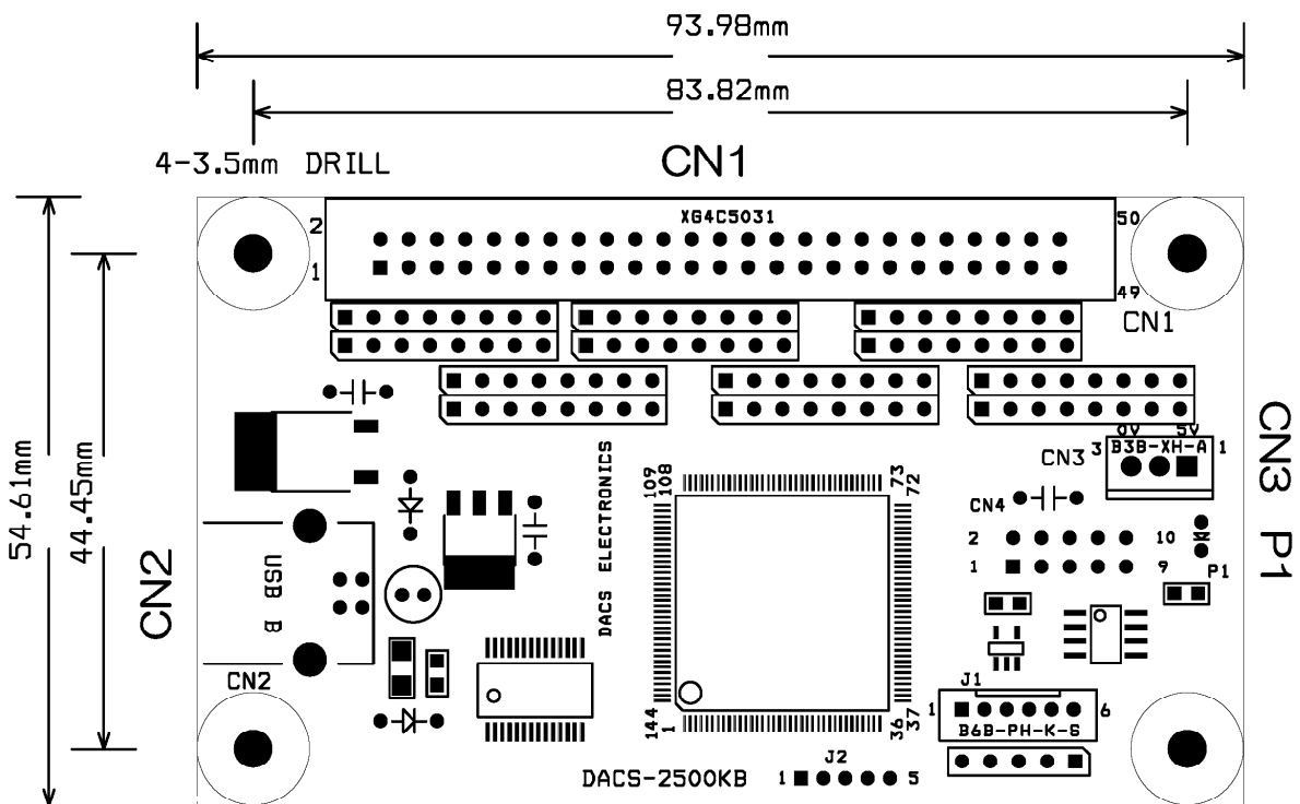
図 1. 2 DACS-2500KB-RSV3 外形図
