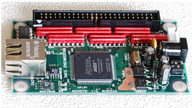
リモートIO基板 RM5500A
